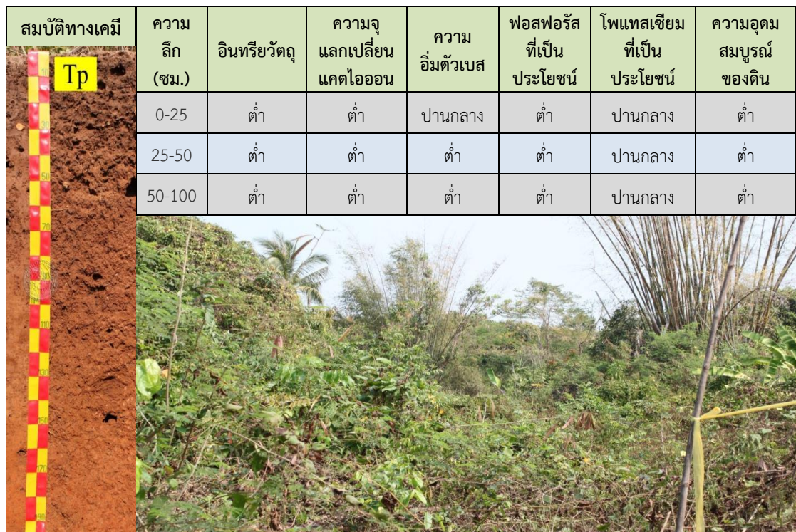
ภาพที่ 1 หน้าตัดดินและคำบรรยายชุดดินธาตุพนม
