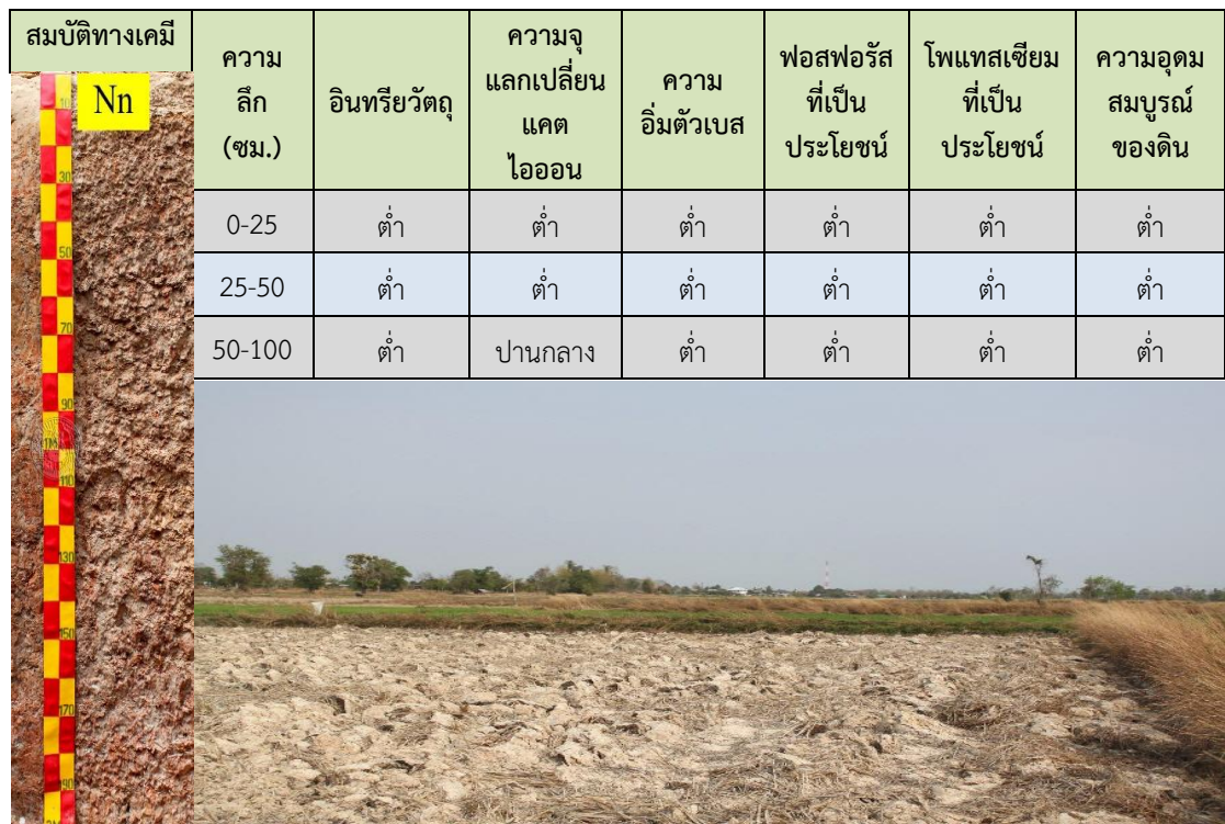
ภาพที่ 2 หน้าตัดดินและคำบรรยายชุดดินนครพนม
