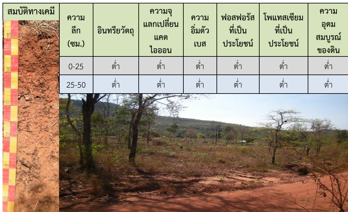
ภาพที่ 5 หน้าตัดดินและคำบรรยายชุดดินวังน้ำเขียว
