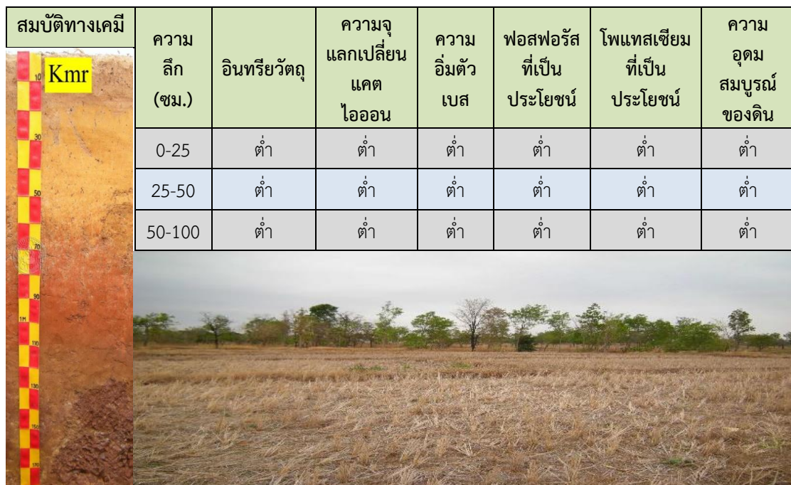
ภาพที่ 3 หน้าตัดดินและคำบรรยายชุดดินเขมราฐ
