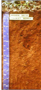
ชุดดินภูเก็ต (Pk)
