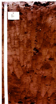
ชุดดินสีคิ้ว (Si)
