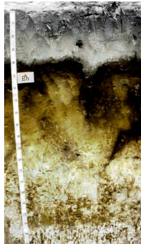
ชุดดินบ้านทอน (Bh)
