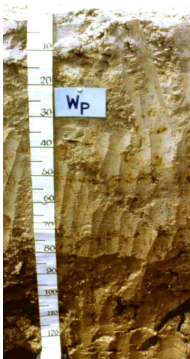
ชุดดินวัลเปียง (Wp)
