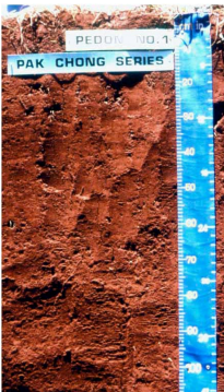
ชุดดินปากช่อง (Pc)
