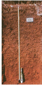
ชุดดินเชียงคาน (Ch)
