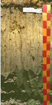
ชุดดินชะอำ (Ca)
