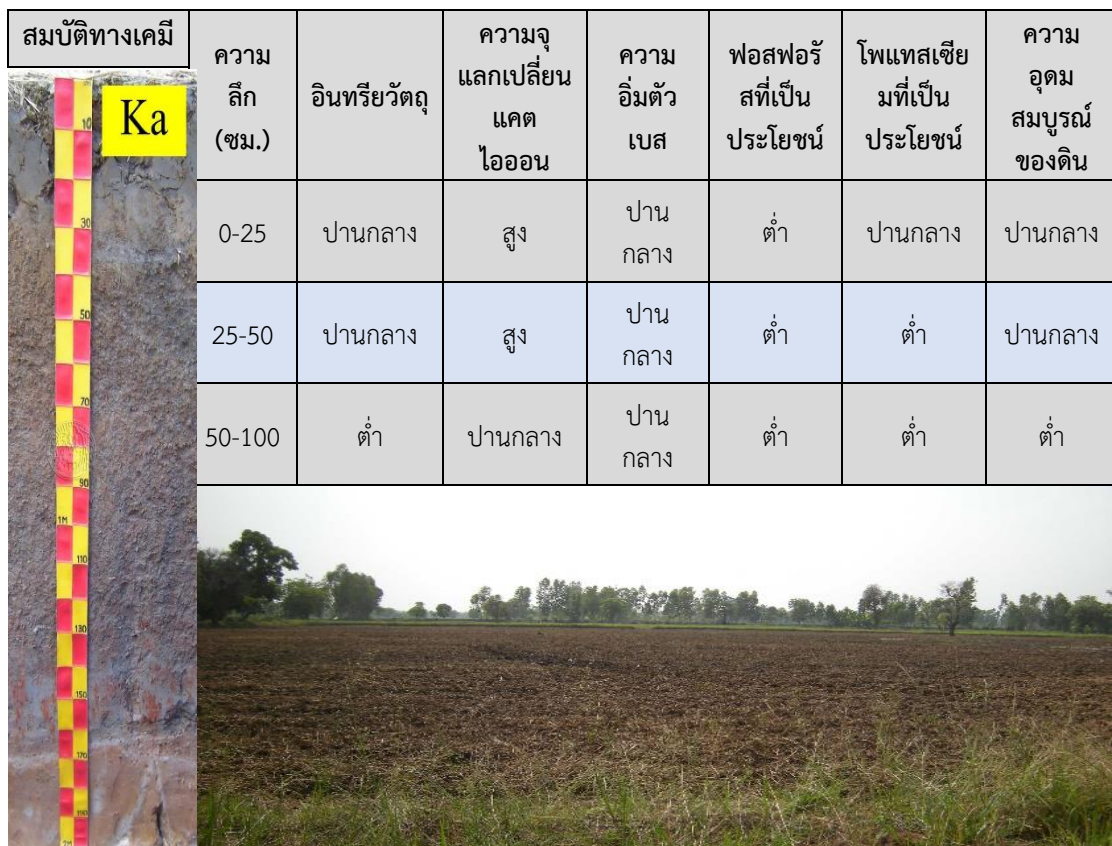
ภาพที่ 1 หน้าตัดดินและคำบรรยายชุดดินกันทรวิชัย
